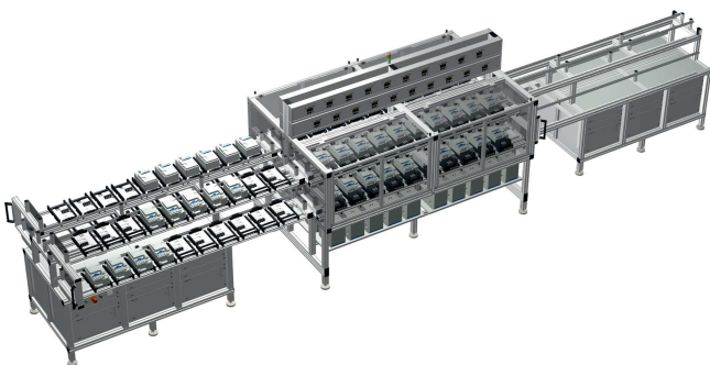
Sistema de Ensayo Automático con MSVT para el ensayo eficiente de 48 contadores monofásicos
