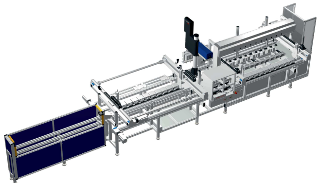
Sistema de Ensayo Completamente Automático con varios pasos / estaciones de ensayo específicos del cliente
