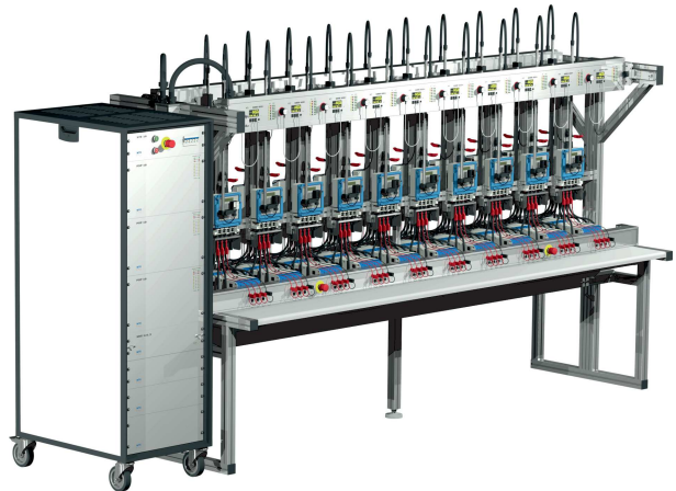
Sistema de Ensayo de Contadores con ICT 2.3 para el ensayo de 20 contadores trifásicos sin necesidad de abrir el puente de tensión
